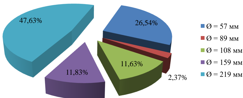
Рисунок 2.3.2.2 – Доли протяжённости участков трубопроводов тепловых сетей котельных МУП «Энергетик» различных диаметров
